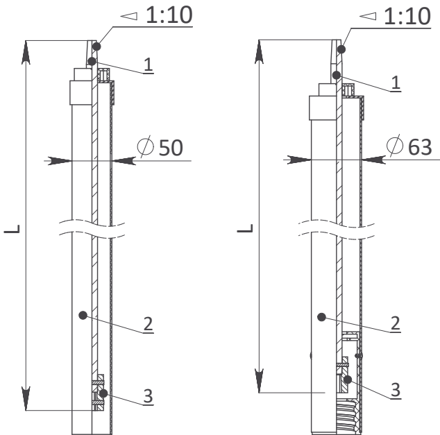
1 – čtvercová tyč 14x14 mm, 2 – ochranná trubka soupravy, 3 – litinová spojka, L – Skutečná délka
